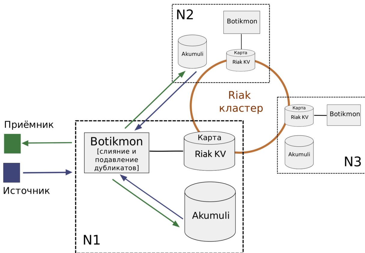
Рис. 1. Архитектура распределённого хранилища
