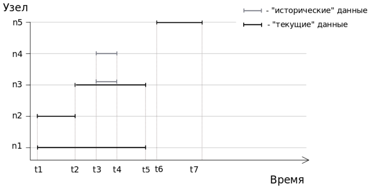
Рис. 2. Пример карты распределения данных одного датчика по узлам
