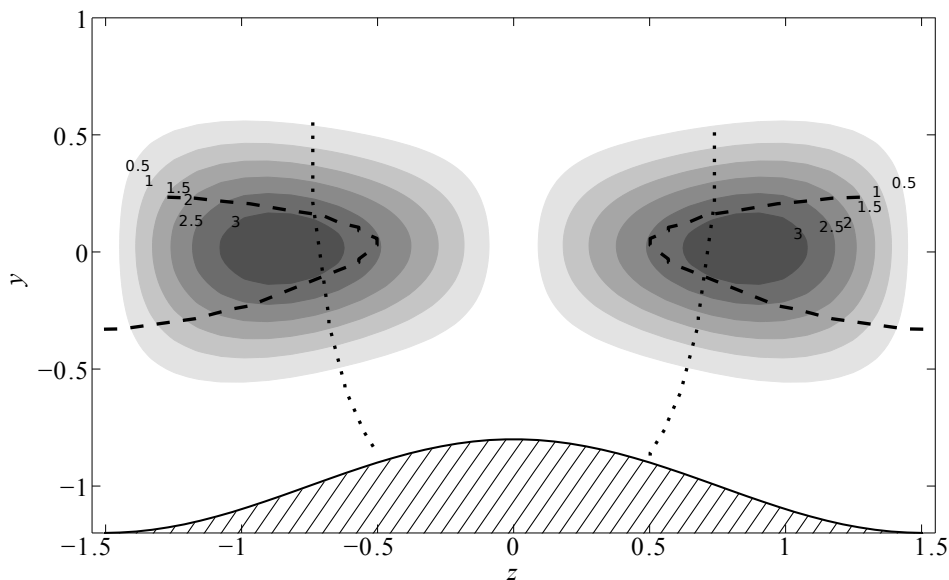
Рис. 15.14. Линии уровня модуля продольной компоненты скорости ведущей моды и точки, в которых \partial^2 U / \partial z^2 = 0 (пунктир) и U = c (штриховые линии), при L = 3.012 , \varepsilon = 0.4 , \rho = 2 и Re = Re_L .
