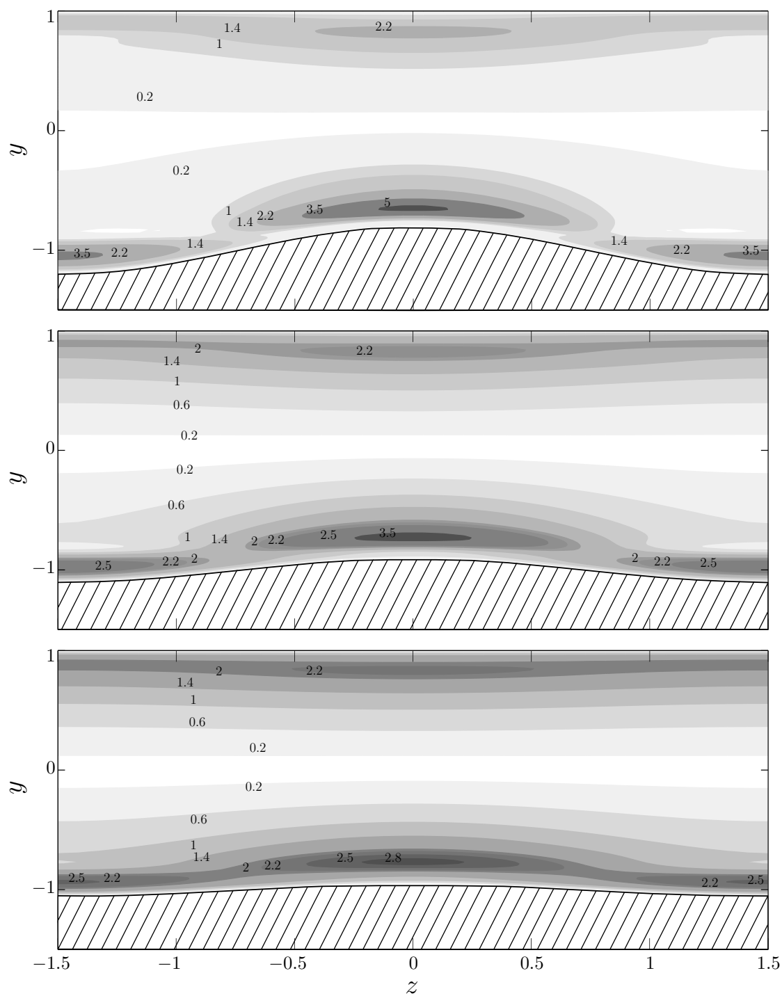
Рис. 15.9. Линии уровня модуля продольной компоненты скорости нейтрально устойчивой моды симметрии I , обеспечивающей \text{Re}_L^I в оребренном канале с L = 3 и \rho = 2 , при трех значениях \varepsilon = 0.4, 0.2, 0.1 .
