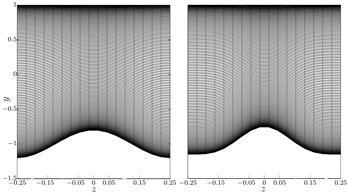
Рис. 13.1. Поперечное сечение канала (один период) при L = 0.5 , \varepsilon = 0.4 и \rho = 2 (слева) и \rho = 4 (справа) и соответствующие сетки с числом узлов m_r \times m_s = 140 \times 17 .
