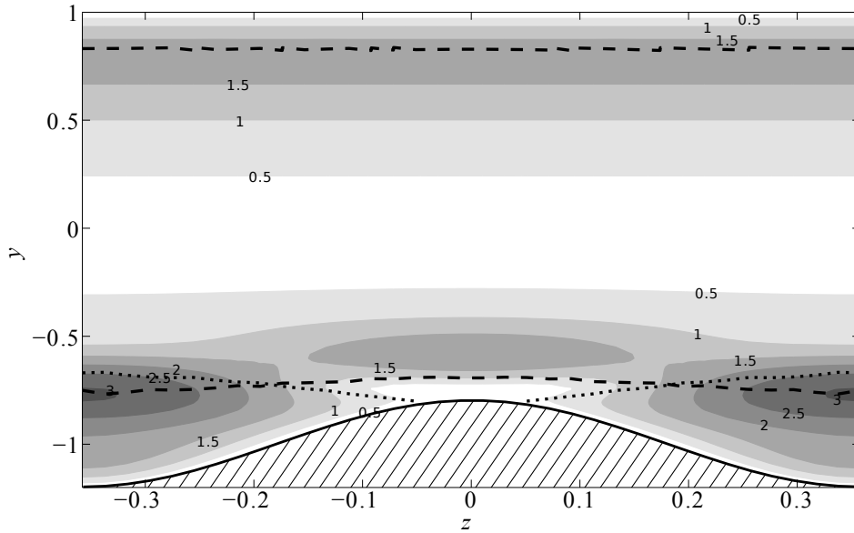
Рис. 15.13. Линии уровня модуля продольной компоненты скорости ведущей моды и точки, в которых \partial^2 U / \partial y^2 = 0 (пунктир) и U = c (штриховые линии), при L = 0.716 , \varepsilon = 0.4 , \rho = 2 и \text{Re} = \text{Re}_L .
