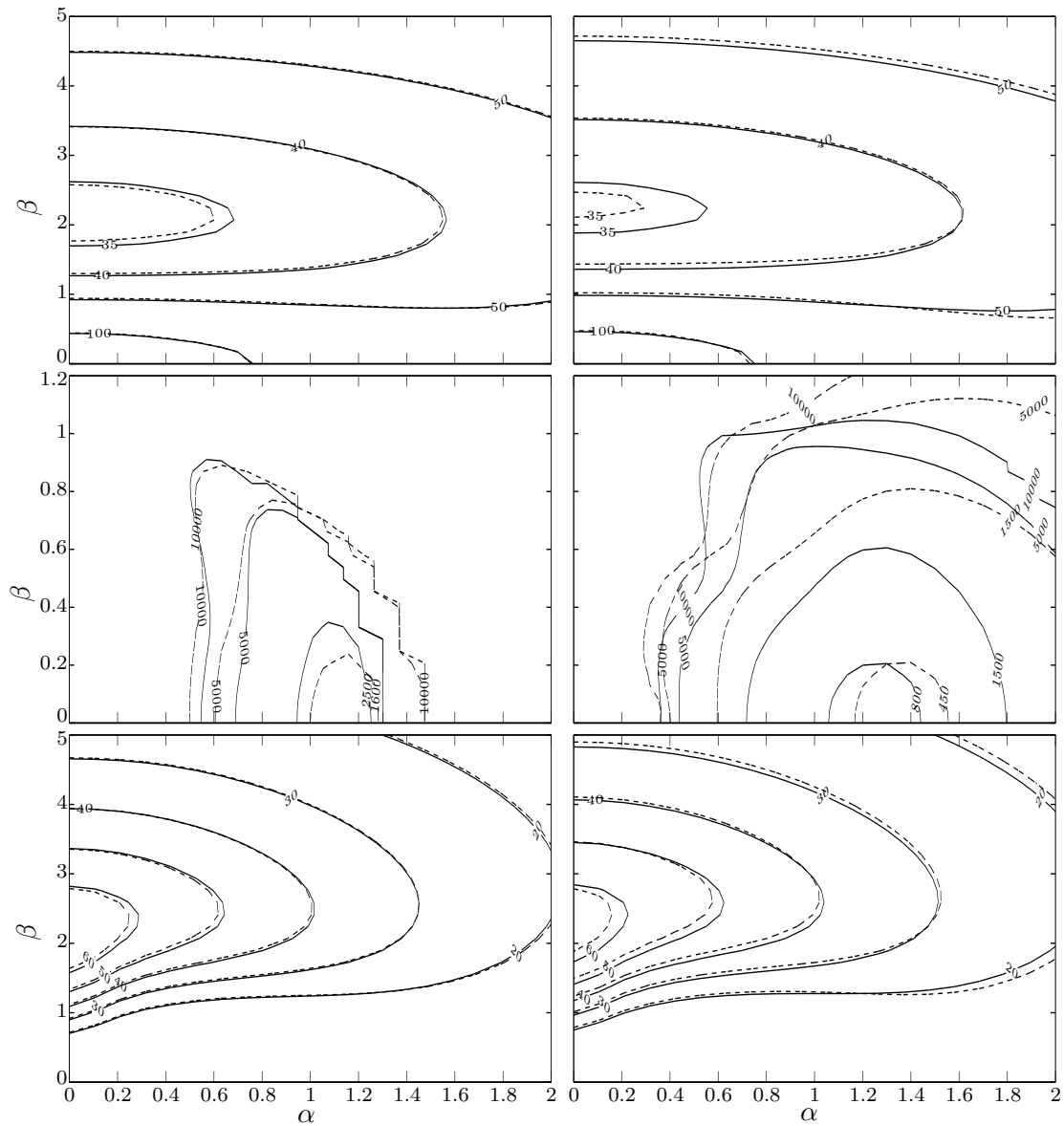
Рис. 14.1. Линии уровня \text{Re}_E^{\alpha\beta} (вверху), \text{Re}_L^{\alpha\beta} (посредине) и \Gamma_{\max}^{\alpha\beta}(400) (внизу) для L = 0.5 и \varepsilon = 0.2 (слева) и 0.4 (справа) при \rho = 2 (—) и 4 (- -).
