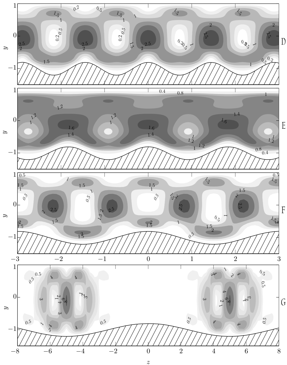
Рис. 15.6. Квадрат модуля проекции скорости критического возмущения, отвечающего Re_E , на плоскость поперечного сечения в оребренном канале при \varepsilon = 0.4 , \rho = 2 и периодах оребрения L = 1.444, 1.836, 3.012 и 10 (D, E, F и G соответственно).
