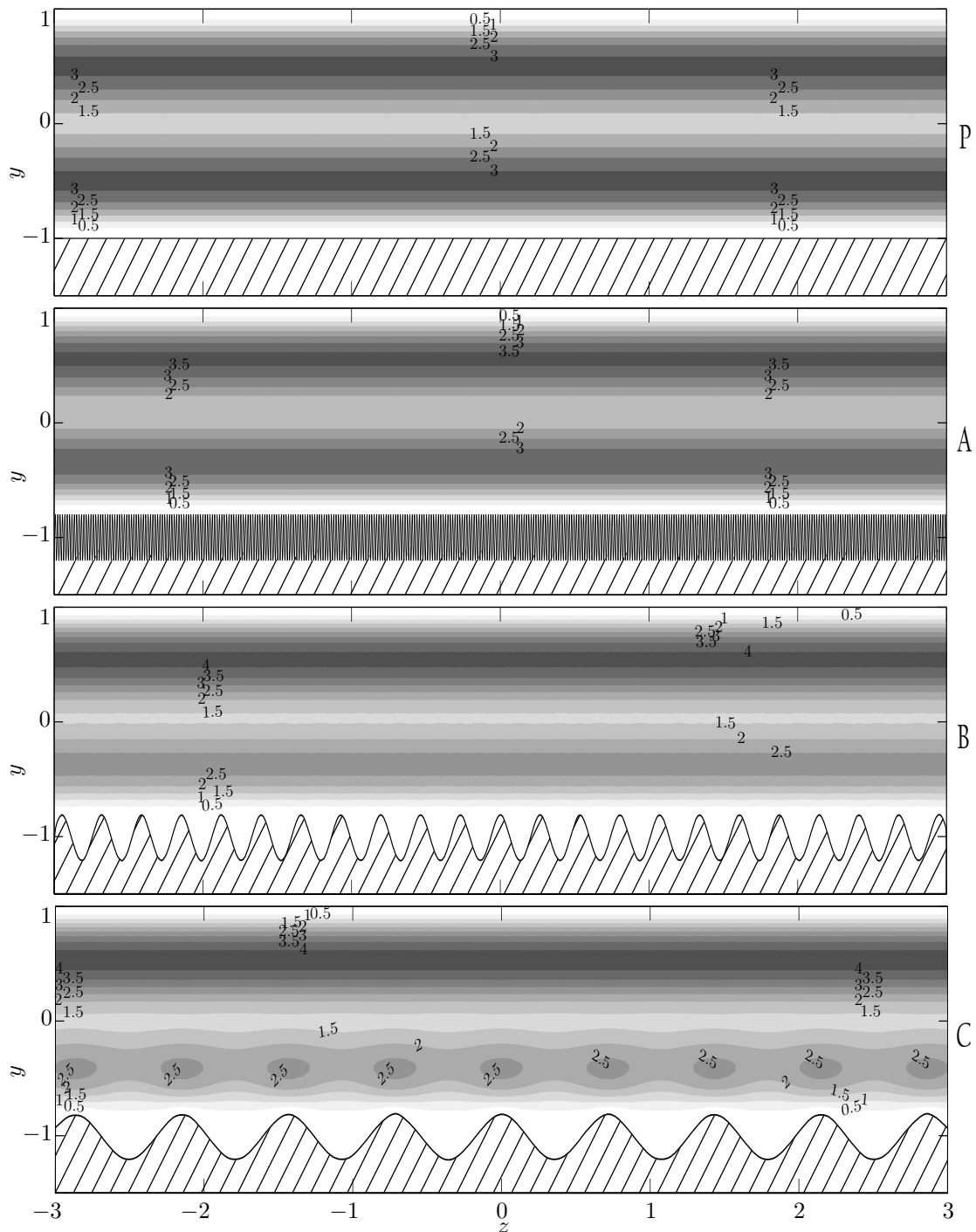
Рис. 15.7. Квадрат модуля полной скорости критического возмущения, отвечающего Re_E , в плоском канале (P) и оребренном канале при \varepsilon = 0.4 , \rho = 2 и периодах оребрения L = 0.016 , 0.268 и 0.716 (A, B и C соответственно).
