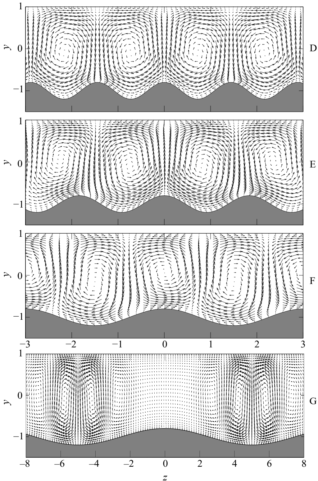
Рис. 15.4. Действительная часть проекции скорости критического возмущения, отвечающего Re_E , на плоскость поперечного сечения в оребренном канале при \varepsilon = 0.4 , \rho = 2 и периодах оребрения L = 1.444 , 1.836 , 3.012 и 10 (D, E, F и G соответственно).
