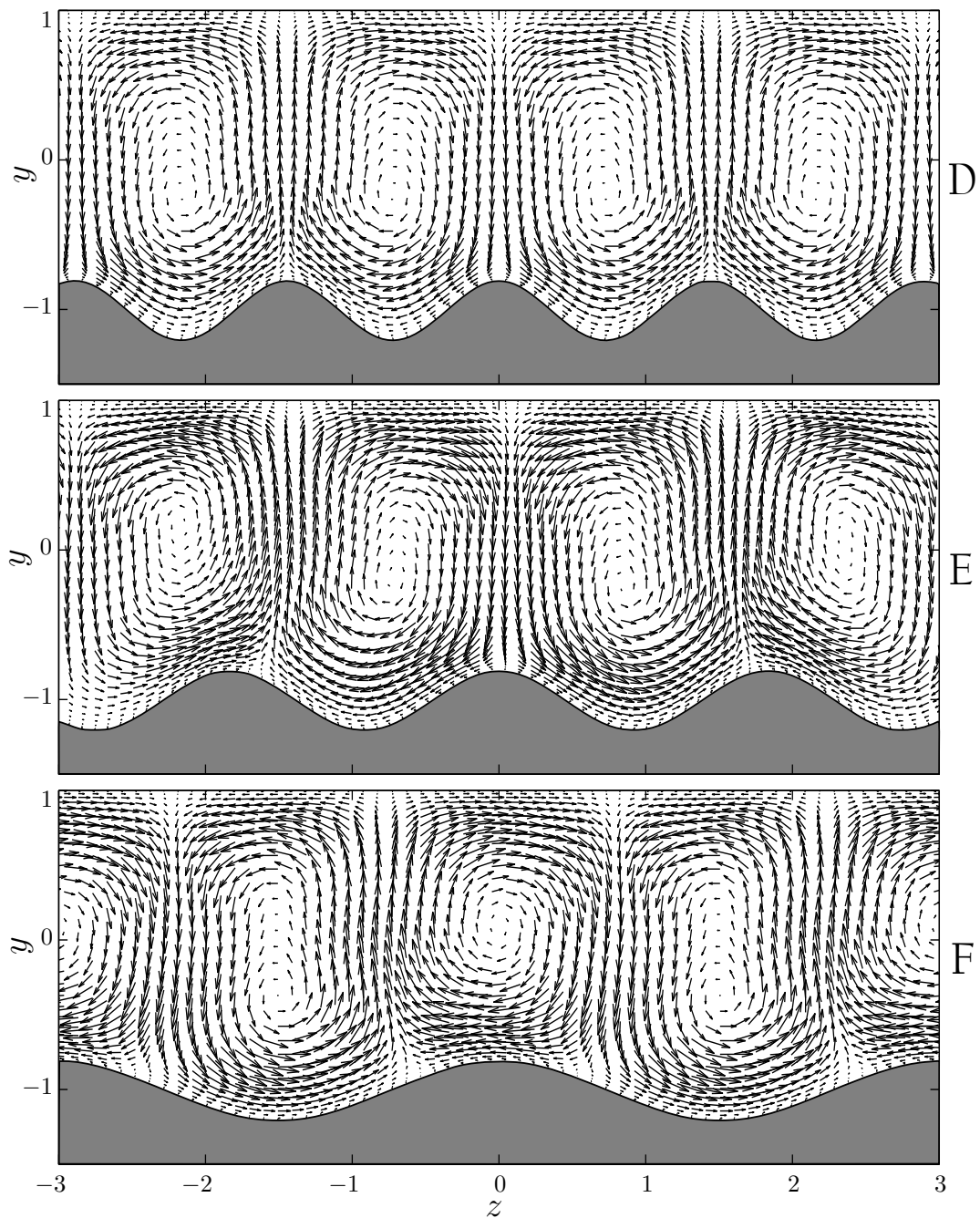
Рис. 16.3. Действительная часть проекции скорости оптимального возмущения на плоскость поперечного сечения в оребренном канале при \varepsilon = 0.4 , \rho = 2 и периодах оребрения L = 1.444 , 1.836 и 3.012 (D, E и F соответственно).
