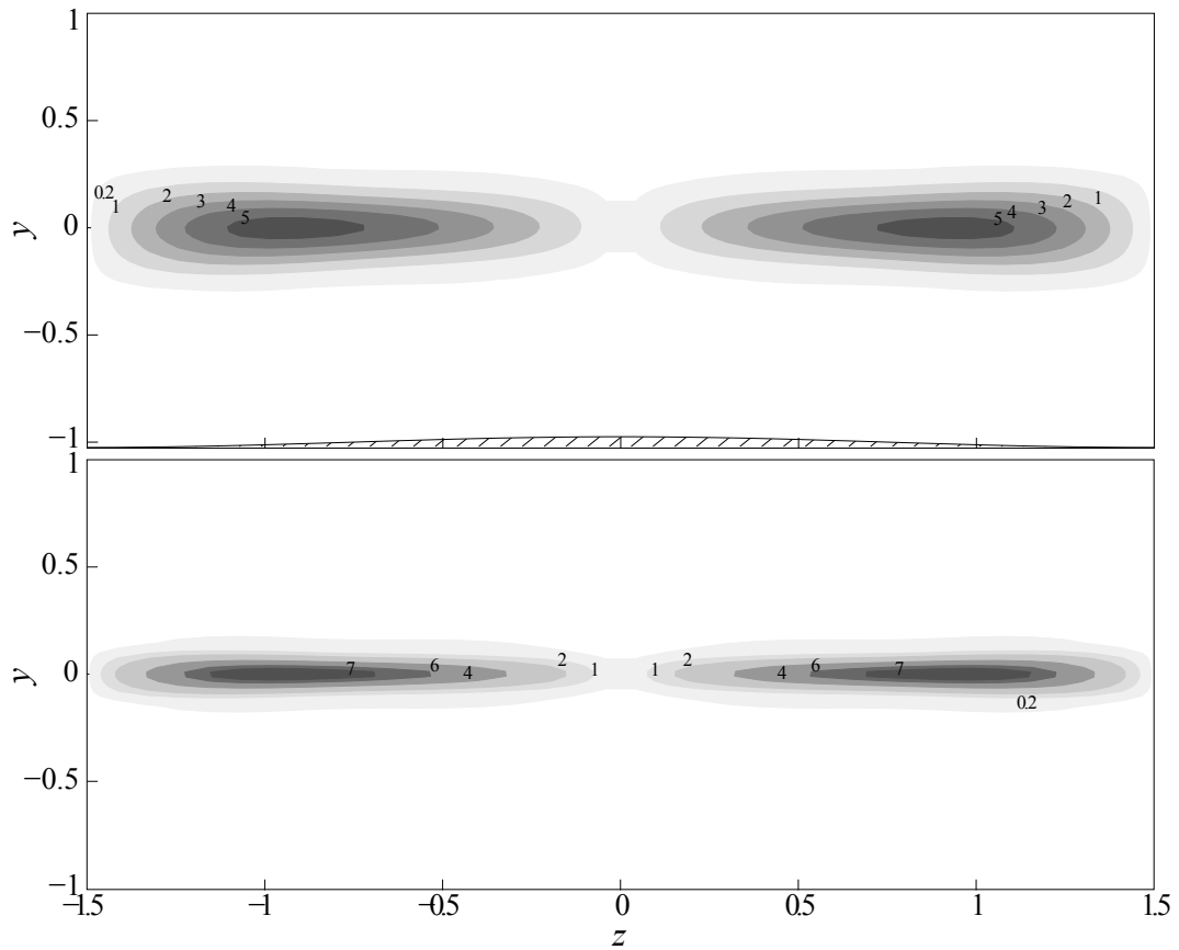
Рис. 15.12. Линии уровня модуля продольной компоненты скорости нейтрально устойчивой моды симметрии II , обеспечивающей \text{Re}_L^{II} в оребренном канале с L = 3 и \rho = 2 , при двух значениях \varepsilon = 0.05, 0.01 .
