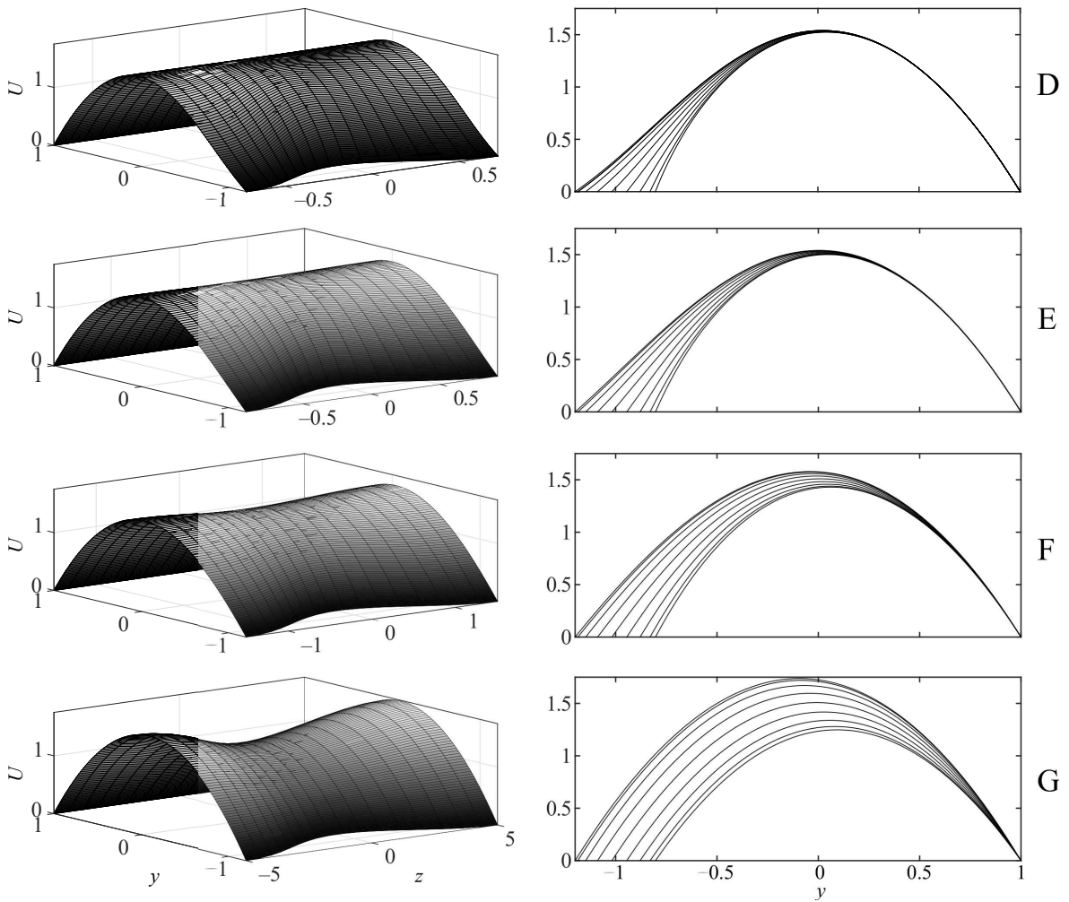
Рис. 13.3. Профиль основного течения в орбренном канале при \varepsilon = 0.4 , \rho = 2 и L = 1.444 , 1.836 , 3.012 и 10 (D, E, F и G соответственно).
