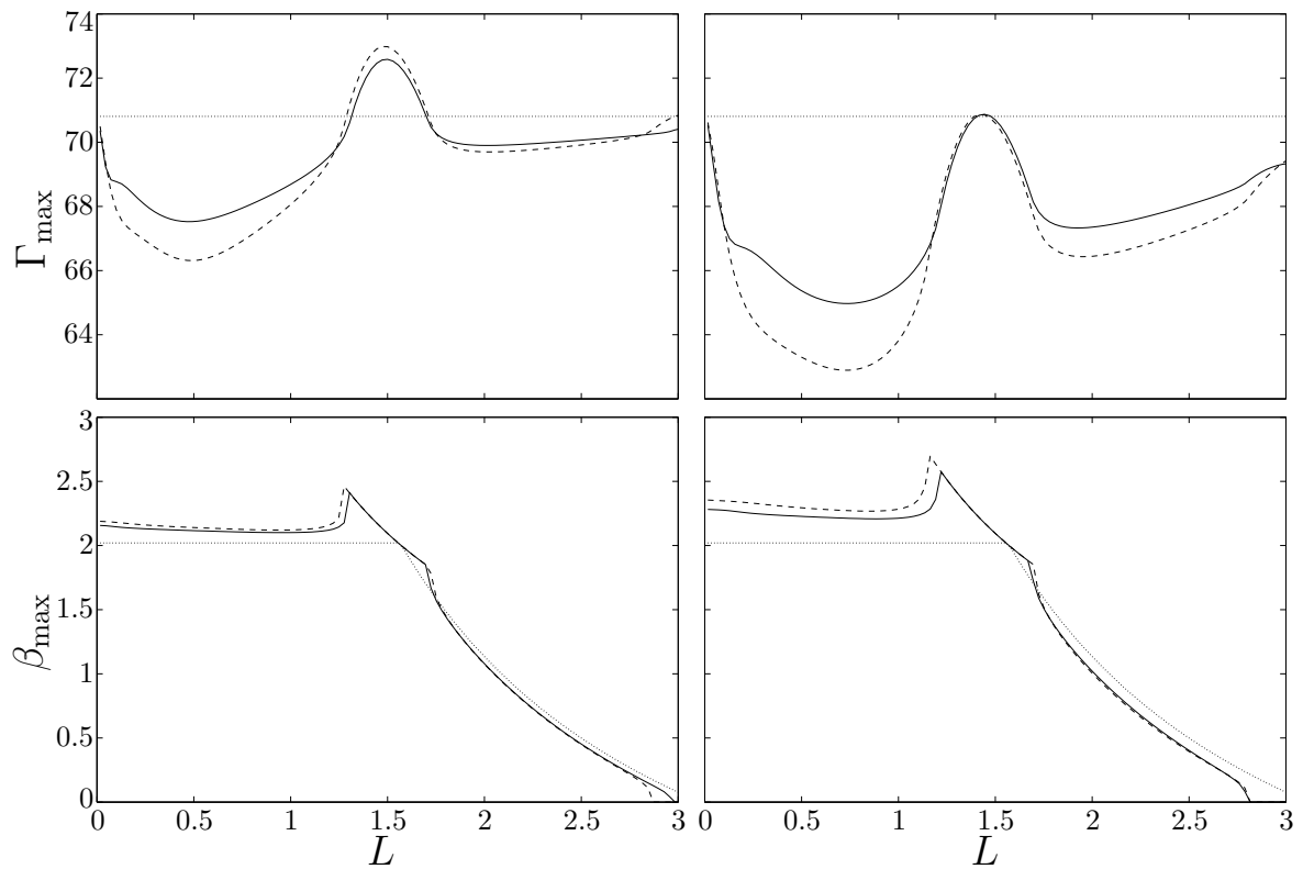
Рис. 16.1. Зависимости \Gamma_{\max} (сверху) и \beta_{\max} (снизу) от периода орбрения для \varepsilon = 0.2 (слева) и 0.4 (справа) при \rho = 2 (—) и 4 (- -).
