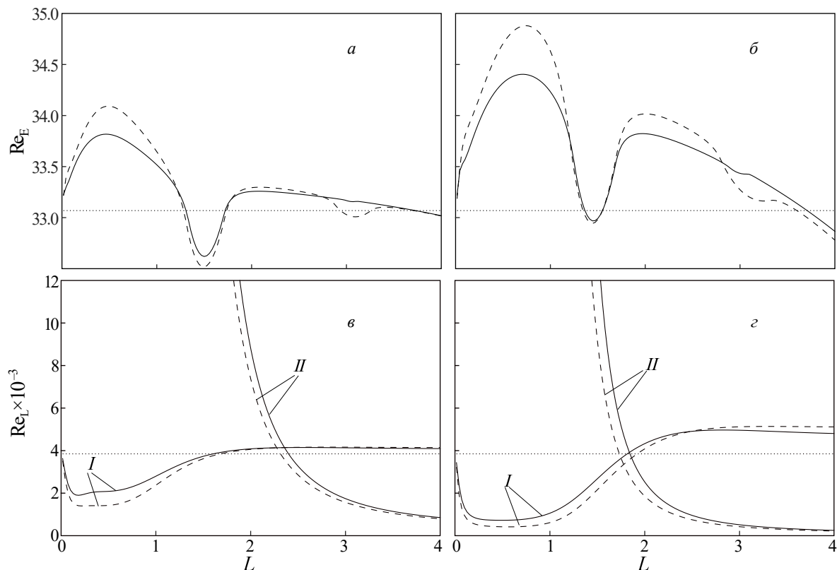
Рис. 15.1. Зависимости Re_E (сверху) и Re_L (снизу) от периода орбления для \varepsilon = 0.2 (слева) и 0.4 (справа) при \rho = 2 (—) и 4 (- -); \widetilde{Re}_E \approx 33.07 , \widetilde{Re}_L \approx 3848 ( \cdots ).
