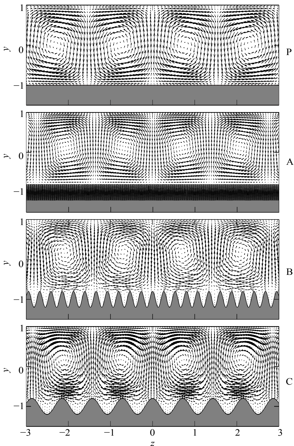
Рис. 15.3. Действительная часть проекции скорости критического возмущения, отвечающего Re_E , на плоскость поперечного сечения в плоском (P) и оребренном канале при \varepsilon = 0.4 , \rho = 2 и периодах оребрения L = 0.016, 0.268 и 0.716 (A, B и C соответственно).
