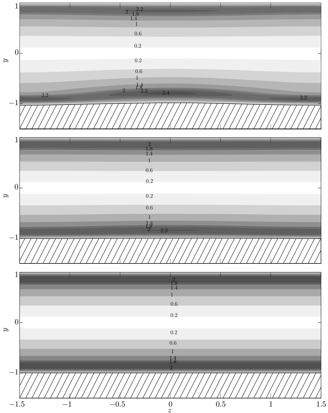
Рис. 15.10. Линии уровня модуля продольной компоненты скорости нейтрально устойчивой моды симметрии I , обеспечивающей \text{Re}_L^I в оребренном канале с L = 3 и \rho = 2 , при двух значениях \varepsilon = 0.05, 0.01 и нейтрально устойчивой моды, отвечающей \widetilde{\text{Re}}_L в плоском канале.
