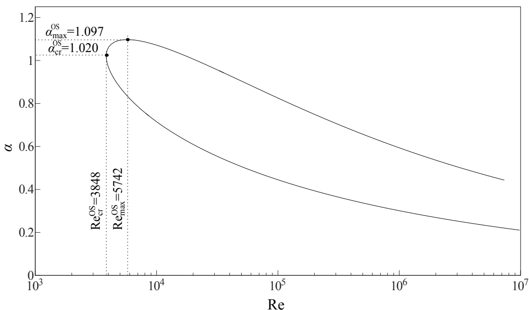
Рис. 6.1. Нейтральная кривая проблемы Орра–Зоммерфельда.
