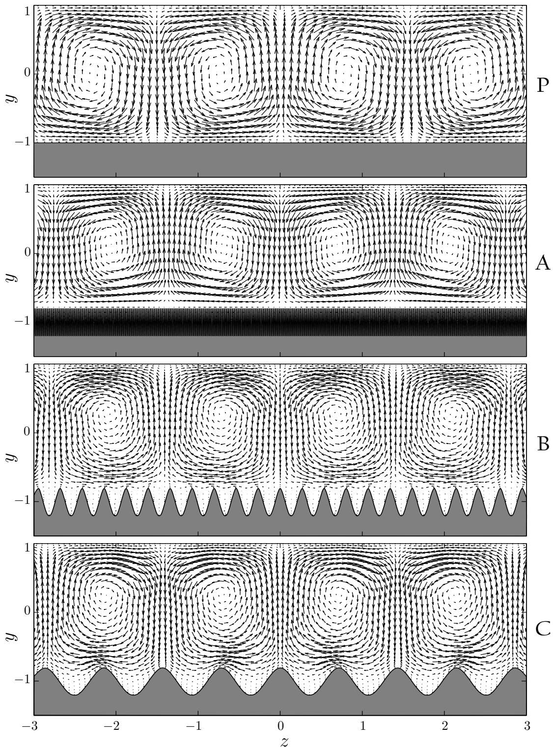
Рис. 16.2. Действительная часть проекции скорости оптимального возмущения на плоскость поперечного сечения в плоском (P) и оребренном канале при \varepsilon = 0.4 , \rho = 2 и периодах оребрения L = 0.016 , 0.268 и 0.716 (A, B и C соответственно).
