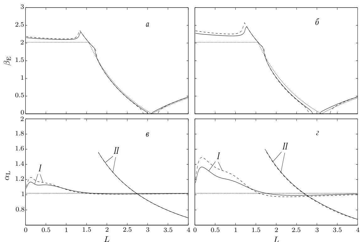
Рис. 15.2. Зависимости \beta_E (сверху) и \alpha_L (снизу) от периода оребрения для \varepsilon = 0.2 (слева) и 0.4 (справа) при \rho = 2 (—) и 4 (- -); \tilde{\beta}_E и \tilde{\alpha}_L ( \cdots ).
