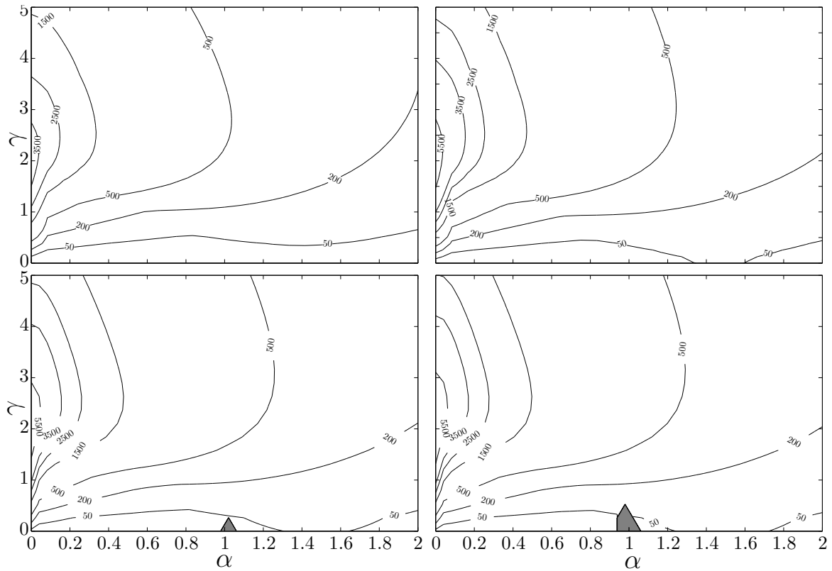
Рис. 14.3. Линии уровня \tilde{\Gamma}_{\max}^{\alpha\gamma}(\text{Re}) для плоского канала, вычисленные при \text{Re} = 3000 (сверху слева), \text{Re} = 3800 (сверху справа), \text{Re} = 3860 (снизу слева) и \text{Re} = 4000 (снизу справа). В темно-серых областях \tilde{\Gamma}_{\max}^{\alpha\gamma}(\text{Re}) = \infty (на двух нижних рисунках).
