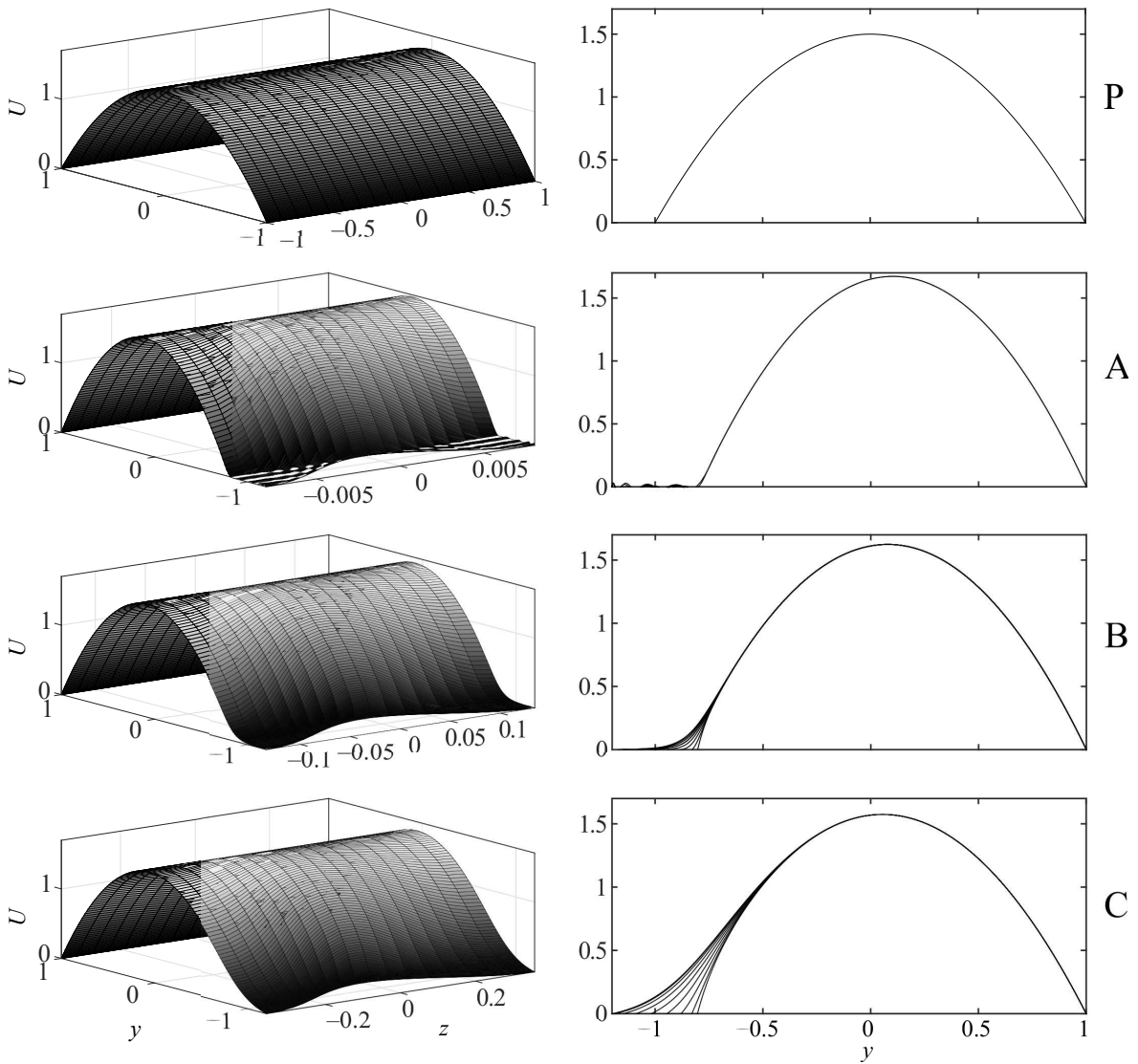
Рис. 13.2. Профиль основного течения в плоском канале (Р) и оребренном канале при \varepsilon = 0.4 , \rho = 2 и L = 0.016 , 0.268 и 0.716 (А, В и С соответственно).
