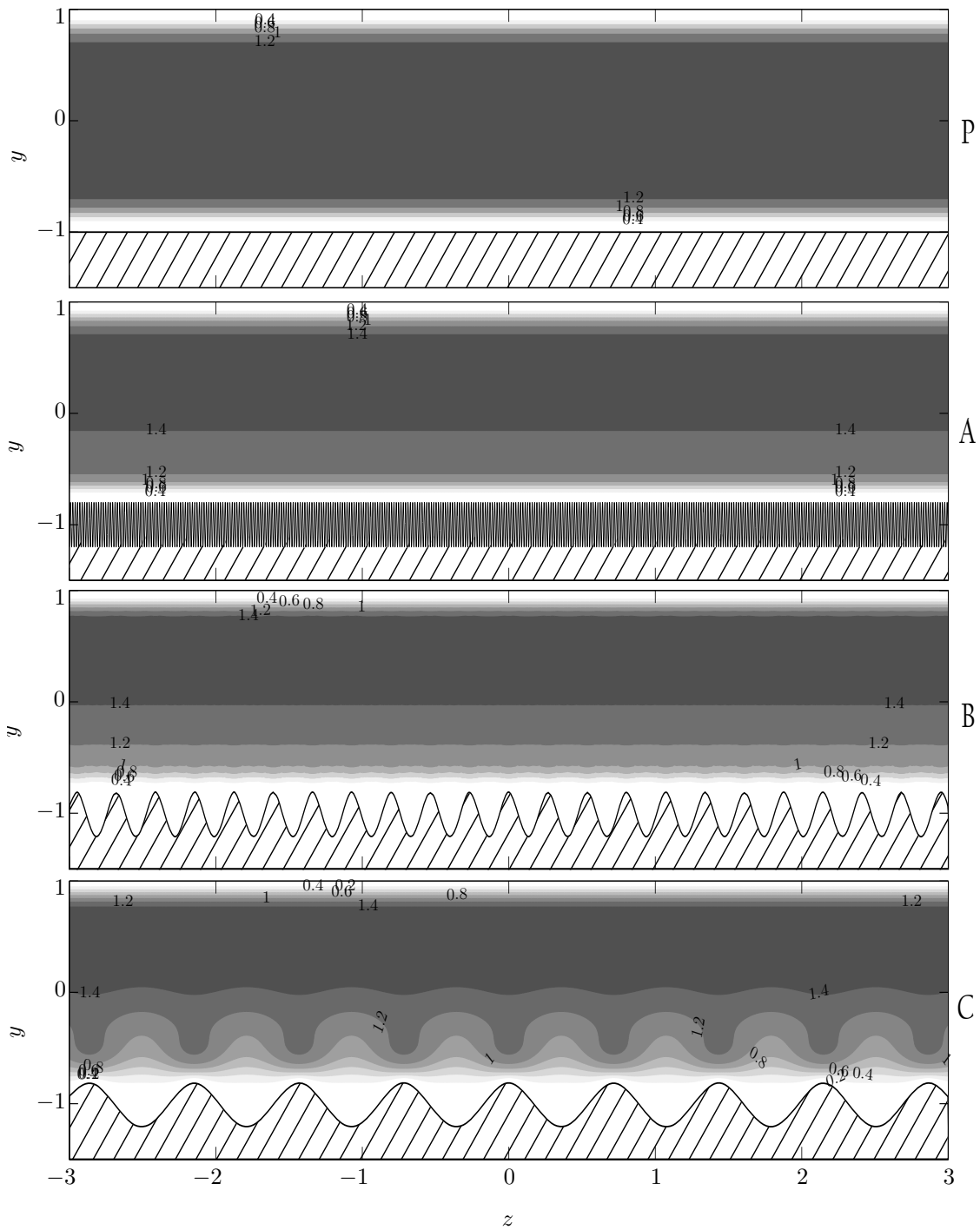
Рис. 15.5. Квадрат модуля проекции скорости критического возмущения, отвечающего Re_E , на плоскость поперечного сечения в плоском канале (P) и оребренном канале при \varepsilon = 0.4 , \rho = 2 и периодах оребрения L = 0.016, 0.268 и 0.716 (A, B и C соответственно).
