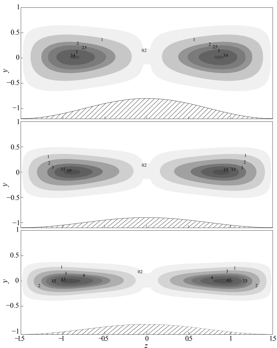
Рис. 15.11. Линии уровня модуля продольной компоненты скорости нейтрально устойчивой моды симметрии II , обеспечивающей \text{Re}_L^{II} в оребренном канале с L = 3 и \rho = 2 , при трех значениях \varepsilon = 0.4, 0.2, 0.1 .
