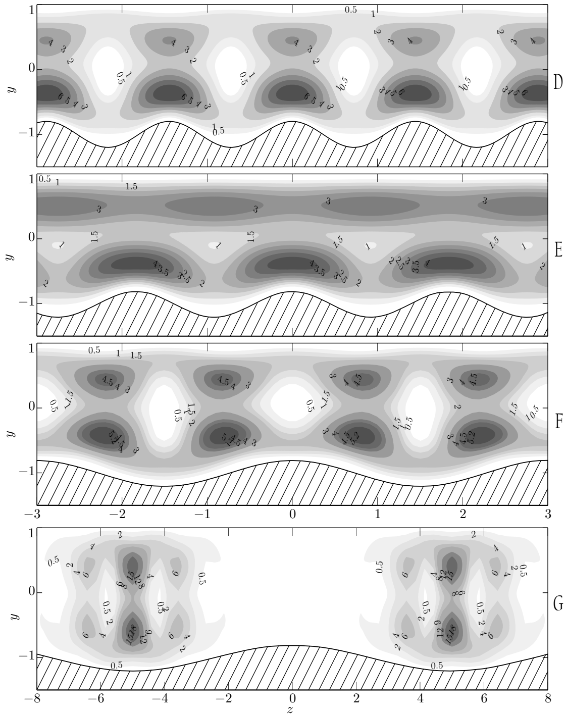
Рис. 15.8. Квадрат модуля полной скорости критического возмущения, отвечающего \text{Re}E , в оребренном канале при \varepsilon = 0.4 , \rho = 2 и периодах оребрения L = 1.444, 1.836, 3.012 и 10 (D, E, F и G соответственно).
