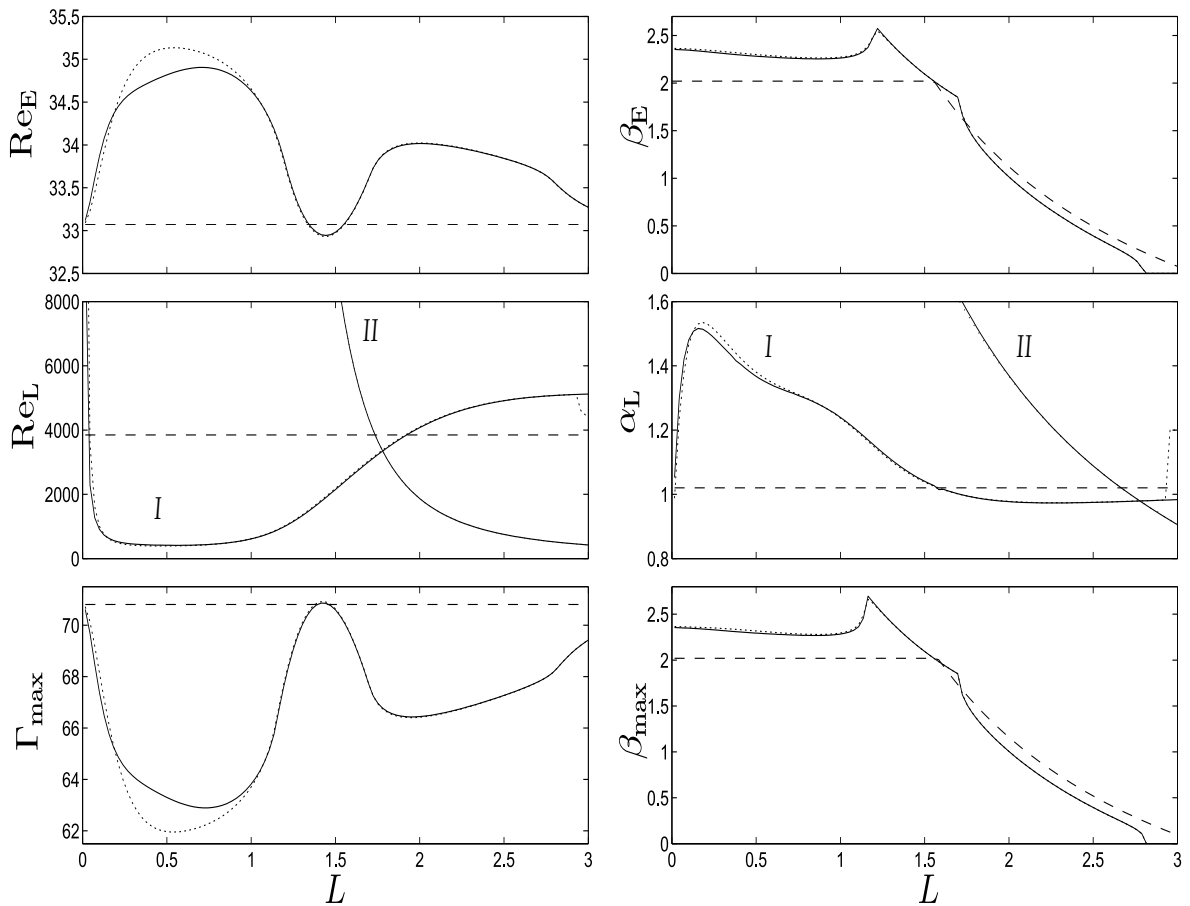
Рис. В.2. Сходимость по шагу сетки при вычислении зависимости характеристик устойчивости от периода оребрения для \varepsilon = 0.4 , \rho = 4 , m_r \times m_s = 80 \times 11 (пунктир) и m_r \times m_s = 140 \times 17 (сплошная линия). Штриховой линией изображены значения характеристик для плоского канала.
