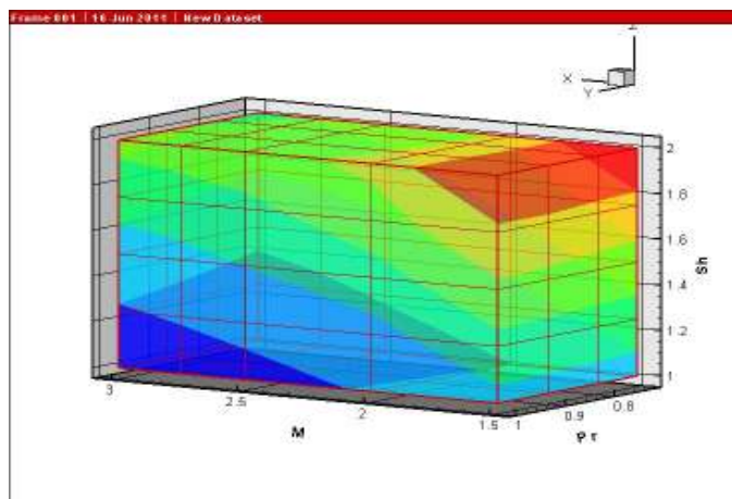
Рис. 6. Зависимость V^*(M_\infty, Pr_\infty, Sh_\infty)
