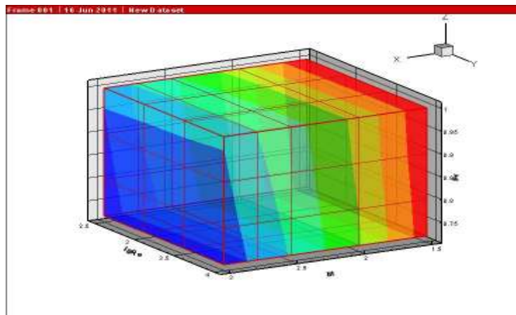
Рис. 5. Зависимость критической скорости повышения нерасчетности от чисел Маха, Рейнольдса и Прандтля
