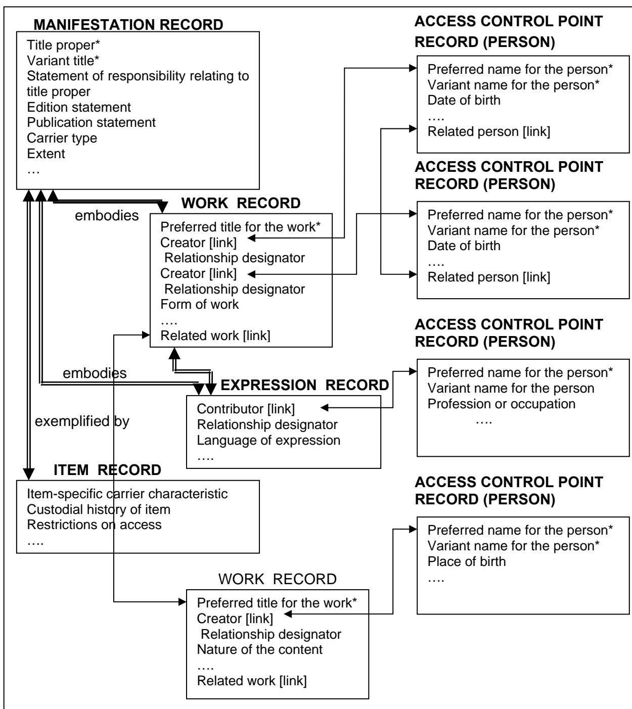
Рис. 4. Реализация RDA в реляционной модели.
