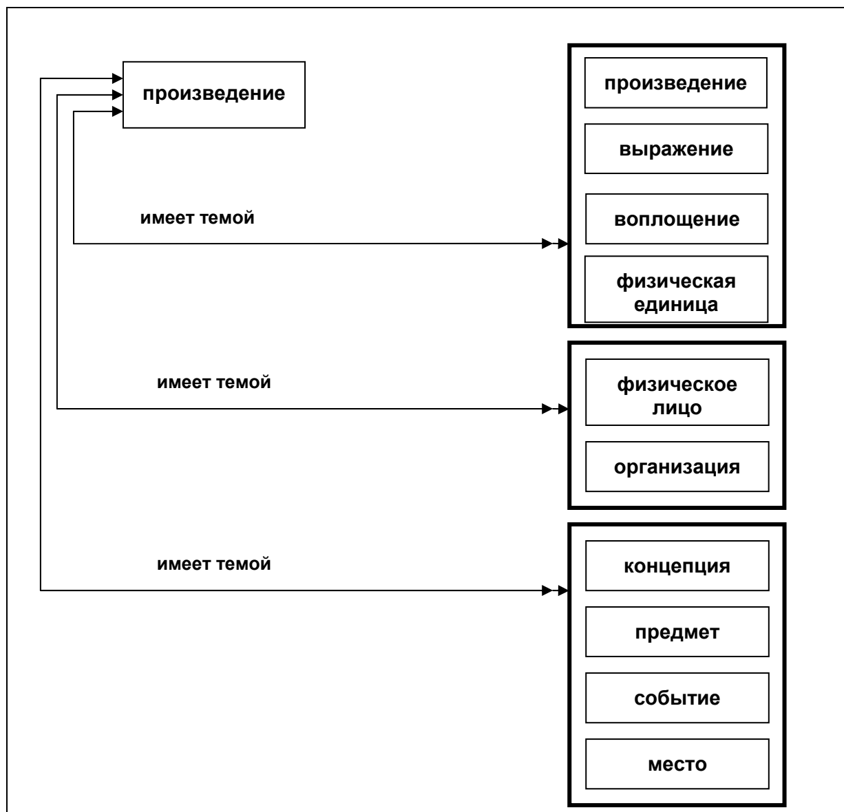
Рис. 3. Группа 3 и связи "тема/содержание".
