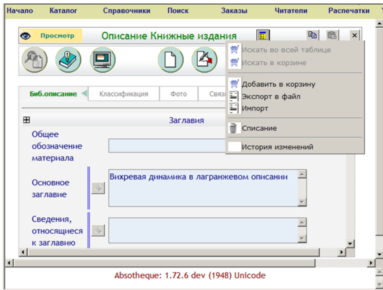
Рис. 7. Выпадающее меню, возникающее при нажатии на значок под названием «Параметры».
