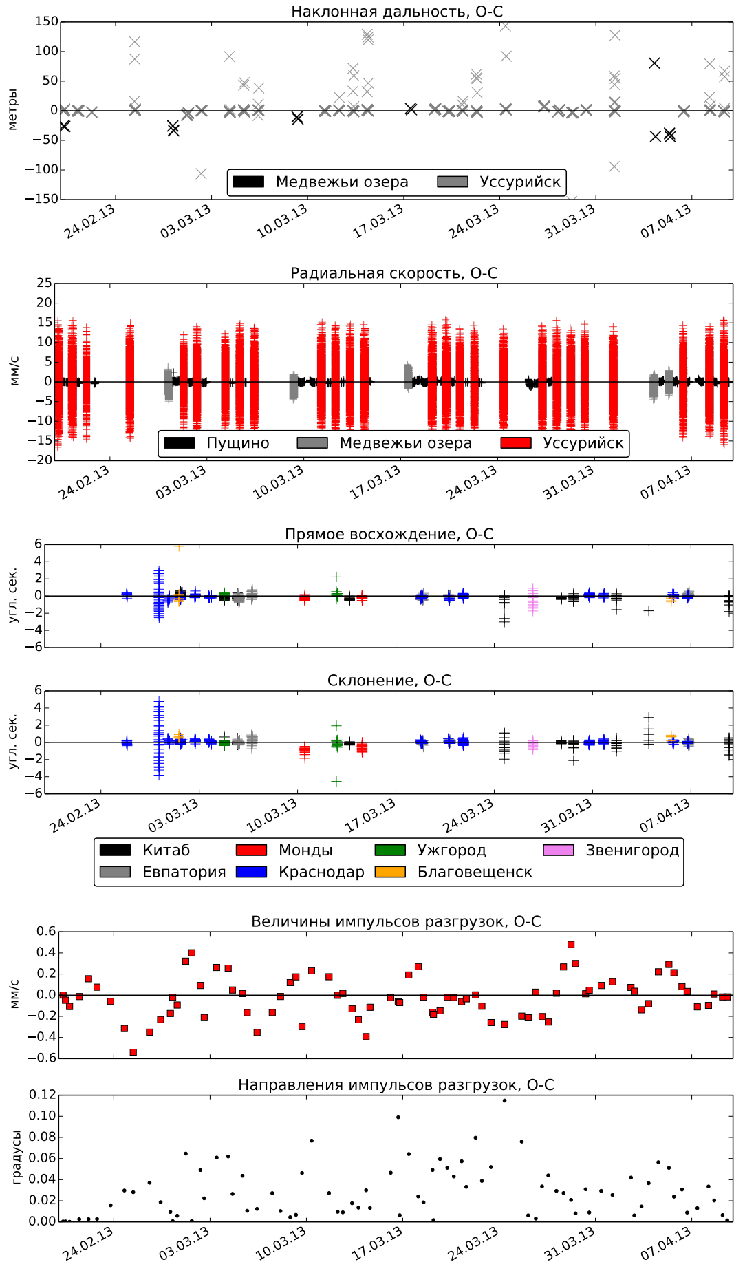
Рис. 7. Рассогласования траекторных измерений КА «Спектр-Р»
