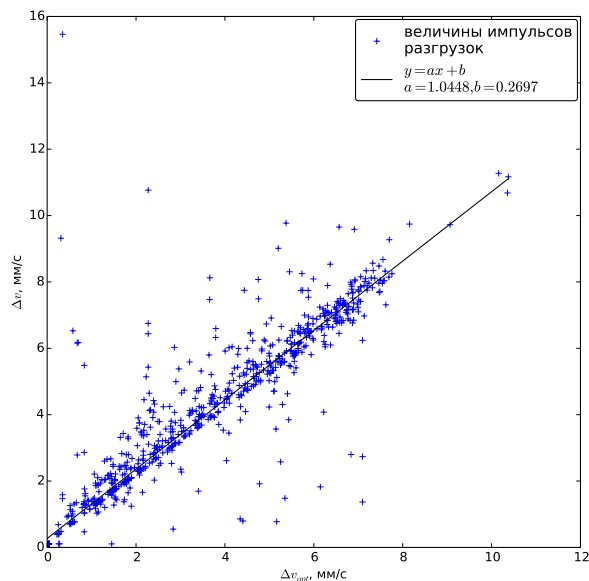
Рис. 3. Соотношение величин импульсов оптимальных и фактических разгрузок 08.2011–09.2013
