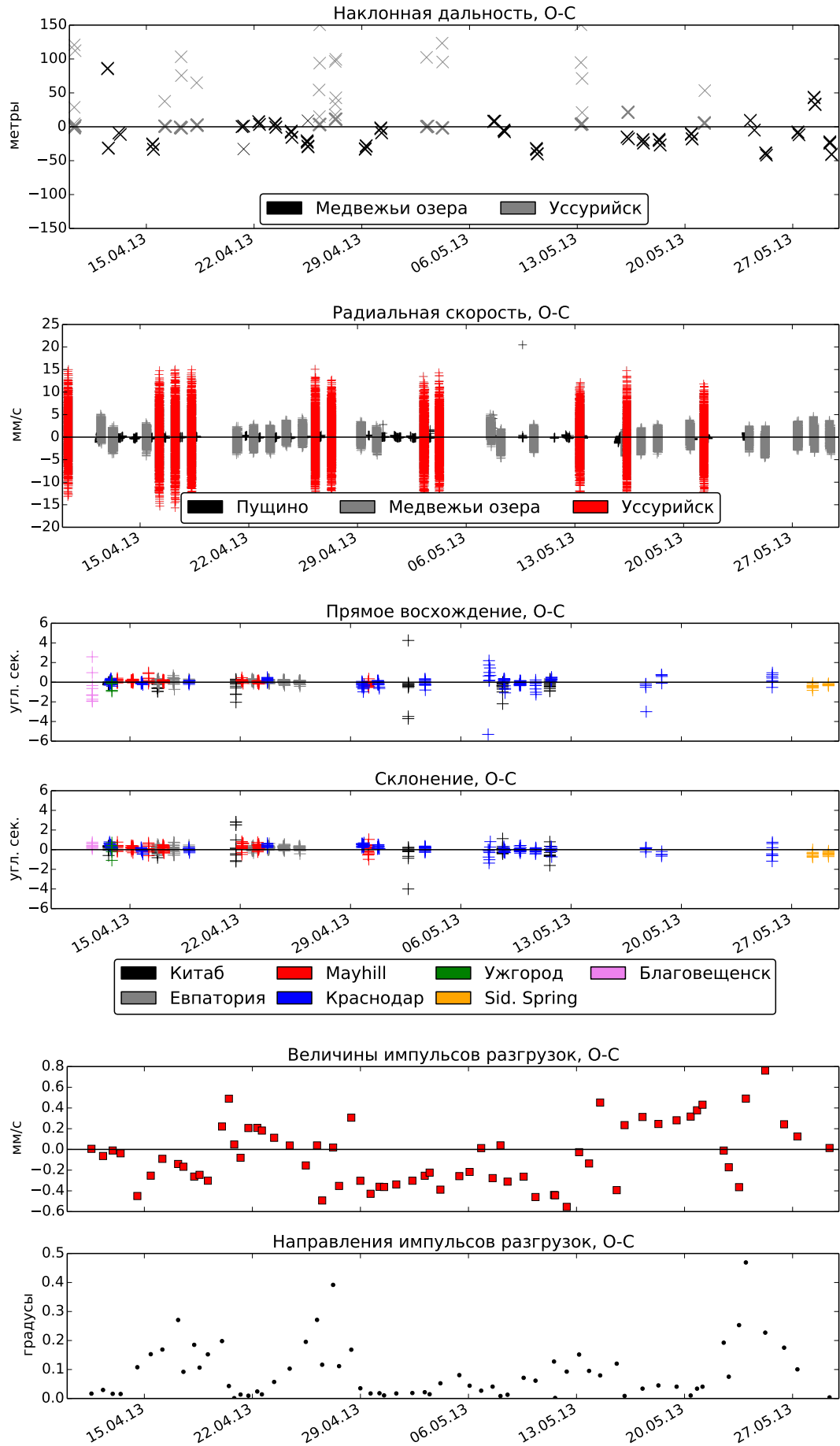
Рис. 8. Рассогласования траекторных измерений КА «Спектр-Р»
