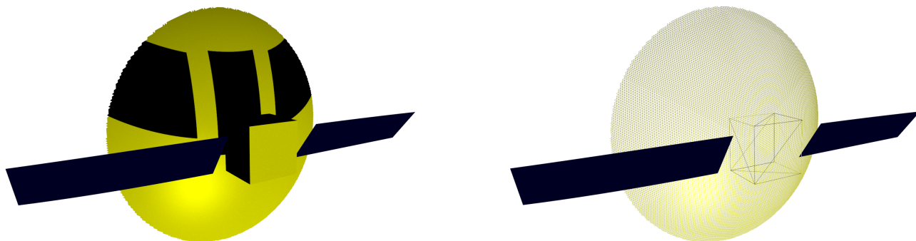
Рис. 2. Модель поверхности КА «Спектр-Р», пример возникающей тени и конечно-элементное представление поверхности КРТ
