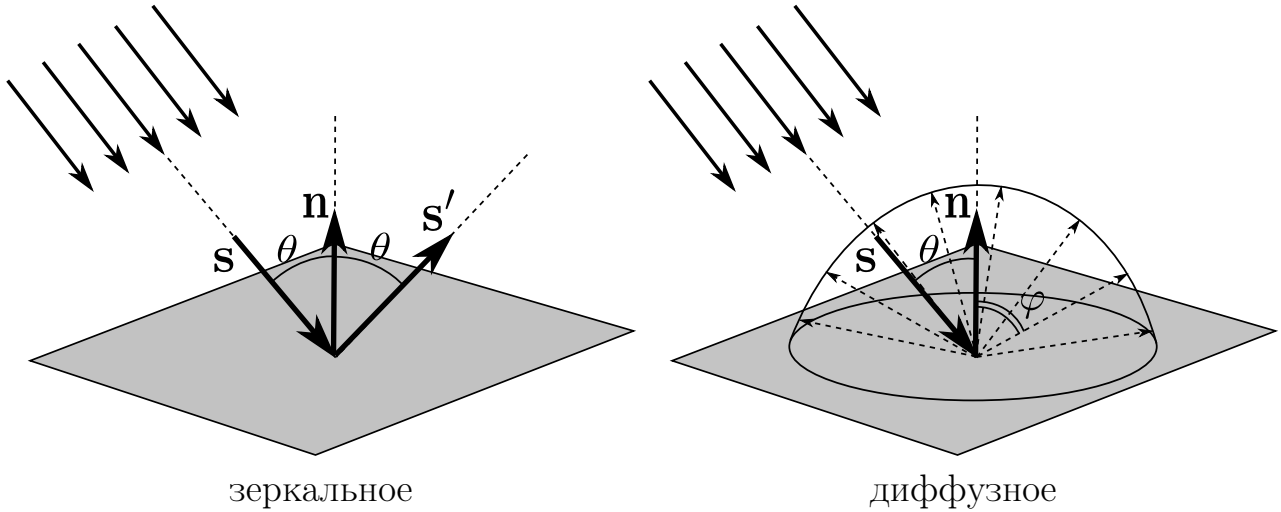
Рис. 1. Отражение света
