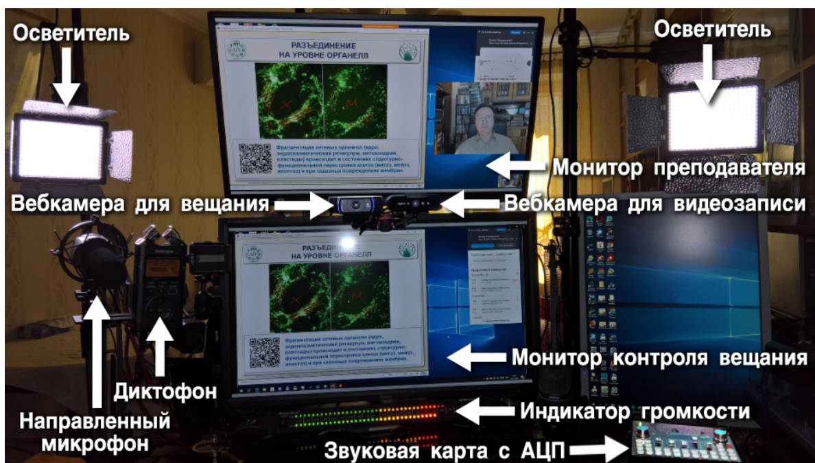
Рис. 4. Оборудование рабочего места преподавателя для онлайн-обучения
