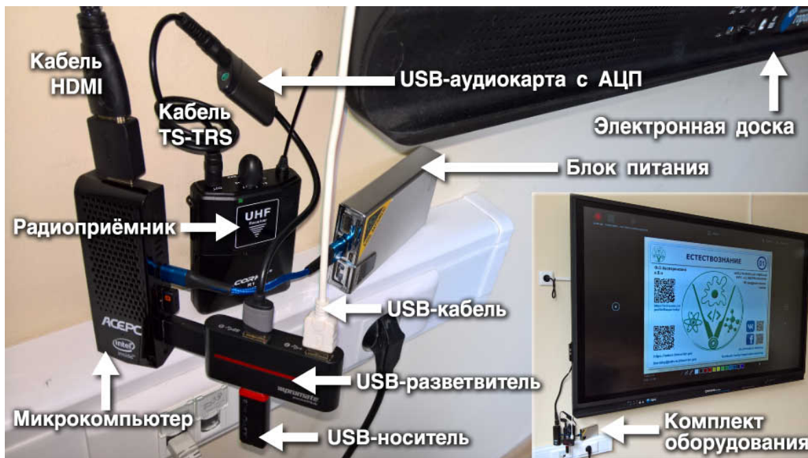
Рис. 3. Микрокомпьютер с дополнительными устройствами ( USB -разветвитель, звуковая карта, радиоприёмник, USB -носитель данных, аккумулятор), подключённый к электронной доске HDMI - и USB -кабелями
