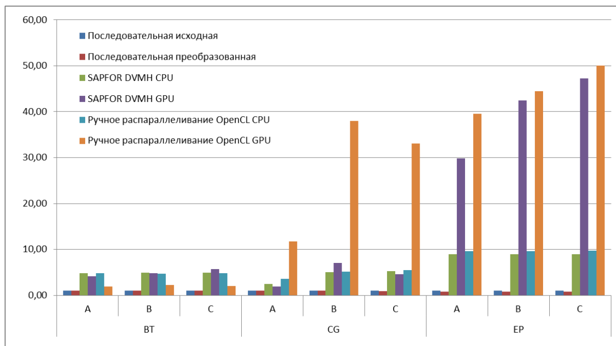
Рис. 2. Ускорение программ из пакета NAS Parallel Benchmarks (NPB)
