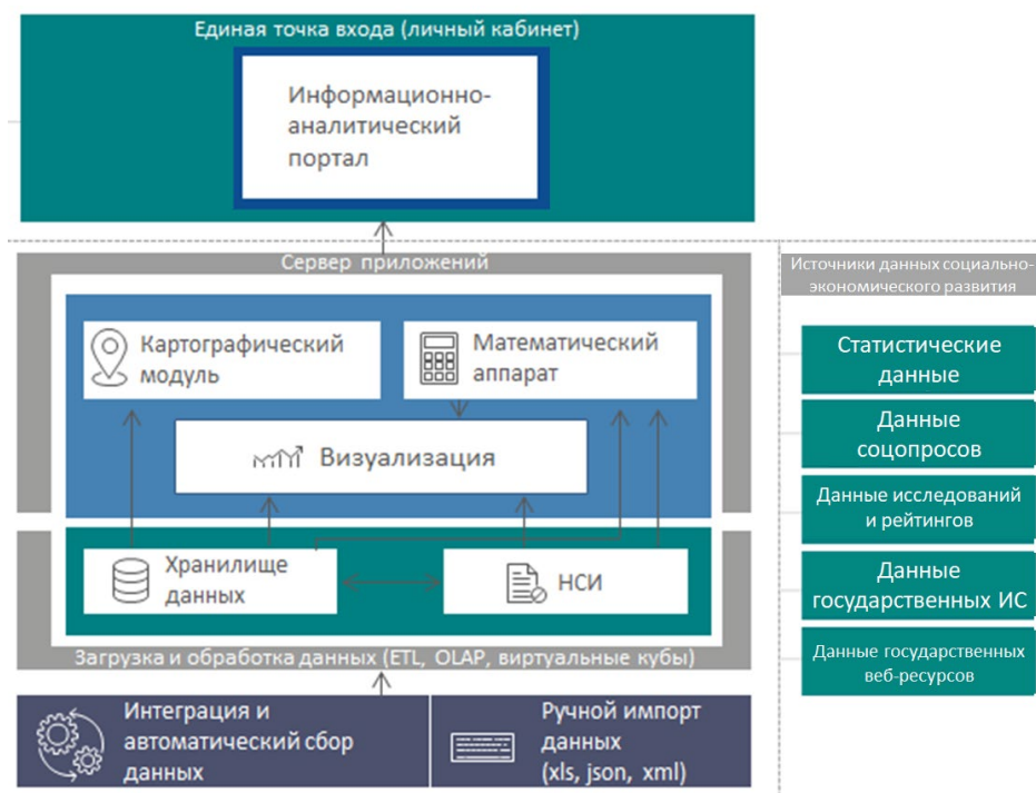
Рис. 1. Архитектура информационно-аналитической системы
