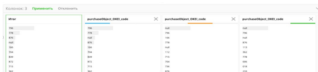
Рис. 5. Интерфейс автоматизированного совмещения столбцов при операции union
