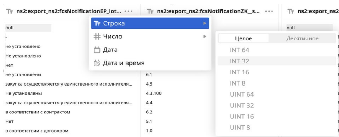
Рис. 6. Интерфейс смены типа данных столбца
