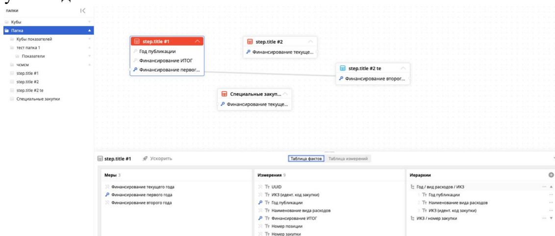
Рис. 7. Интерфейс управления инфологической моделью
