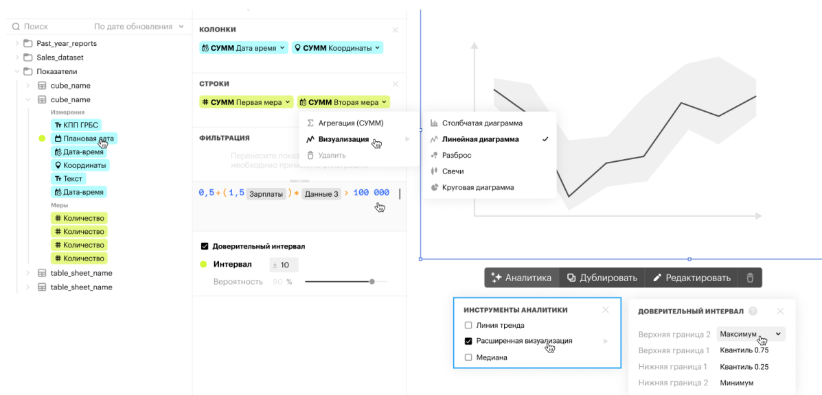
Рис. 9. Интерфейс построения аналитического среза
