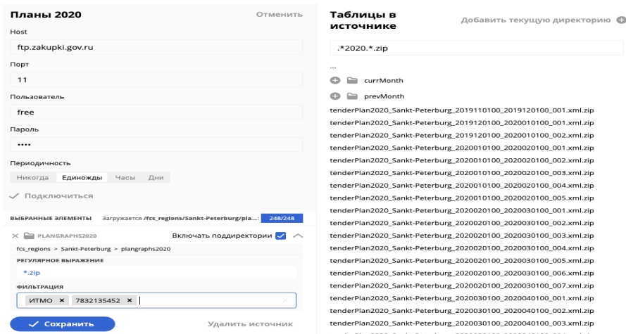
Рис. 2. Интерфейс добавления источника из ЕИС
