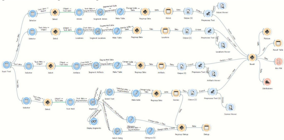
Рис. 3. Нодовая система генерации визуализации сценария
