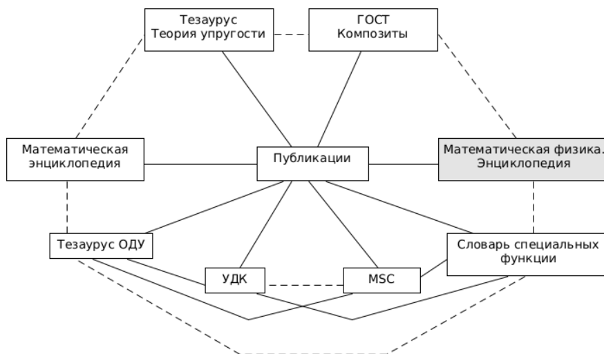
Рис. 4. Схема графа знаний для узла «публикация» (сплошные линии – связи публикации с тезаурусом библиотеки, пунктирные – связи объектов библиотеки с тезаурусом внутри библиотеки)
