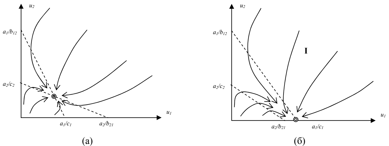
Рисунок П.2. Изменение фазовых траекторий в обществе Западного типа при уменьшении отношения c_1/b_{21} : (а) - начальное состояние, (б) - конечное состояние.
