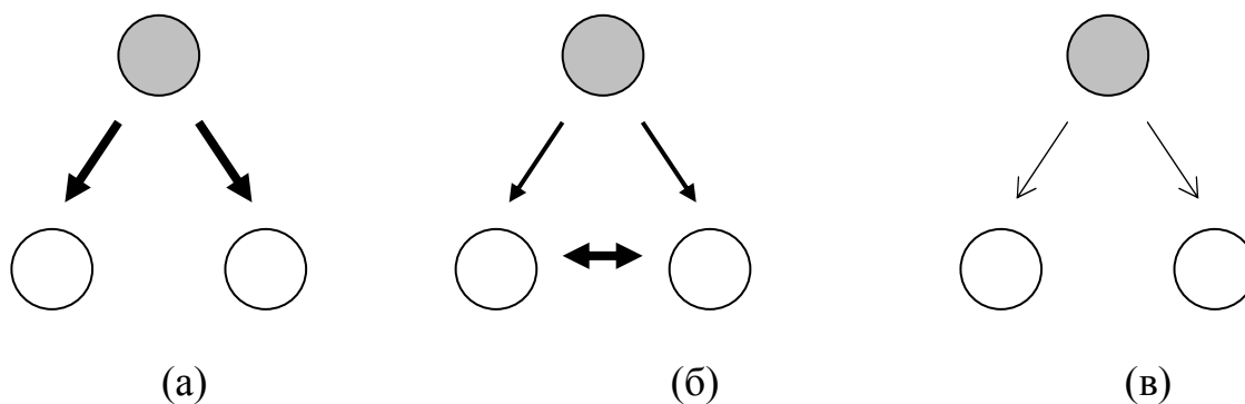
Рисунок П.3. Типовые схемы социального управления на Востоке (а), на Западе (б) и в России (в). (Схемы характеризуют тип взаимодействия центральной власти (круг серого цвета) и управляемых территорий (светлые круги). Толщина стрелок характеризует силу связей между составными частями социума.)
