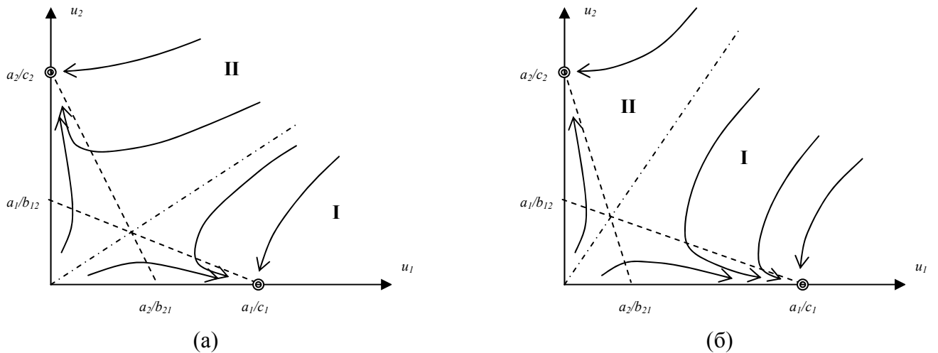
Рисунок П.1. Изменение фазовых траекторий в обществе Восточного типа при уменьшении отношения c_1/b_{21} : (а) - начальное состояние, (б) - конечное состояние.
