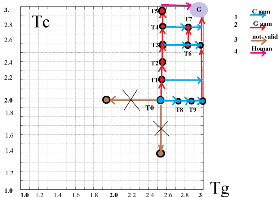
Рис. 10 – Топологическая классификация туров в модели ограниченной задачи четырёх тел в T_i – координатах . 1 – гравманёвры с Каллисто, 2 – гравманёвры с Ганимедом, 3 – «не перспективные» направления, 4 – Гомановский перелёт
