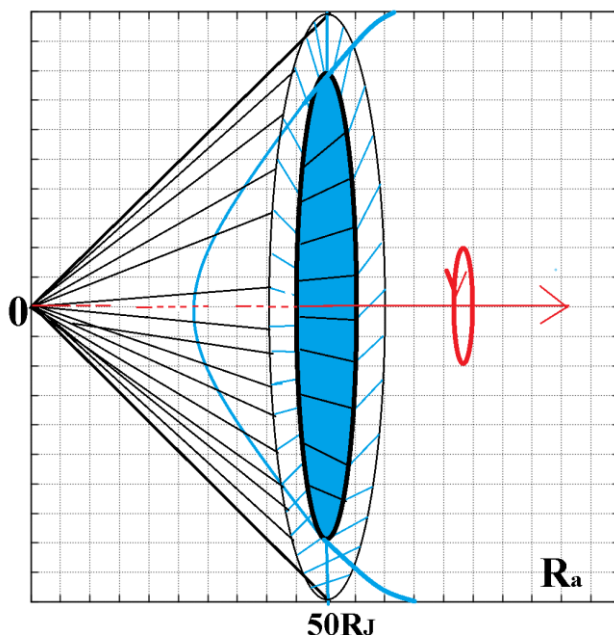
Рис. 4 а) – «Линза» внутри конуса, на которую наматывается траектория КА при гравитационном манёврировании в ограниченной задаче трёх тел
