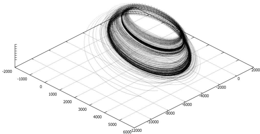
Рис.4 б) – «Перевернутая» вертикально на среднюю плоскость системы Юпитера «линза» внутри конуса, на которую наматывается траектория КА.
