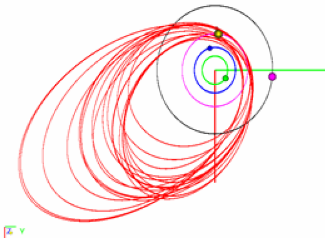
Рис. 22 – Типовой фрагмент манёврирования КА перед посадкой на Ганимед [1–5]. Показаны орбиты КА и спутников Юпитера Ио, Европа, Ганимед, Каллисто
