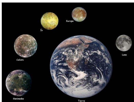
Рис. 7 – Семья Юпитера
