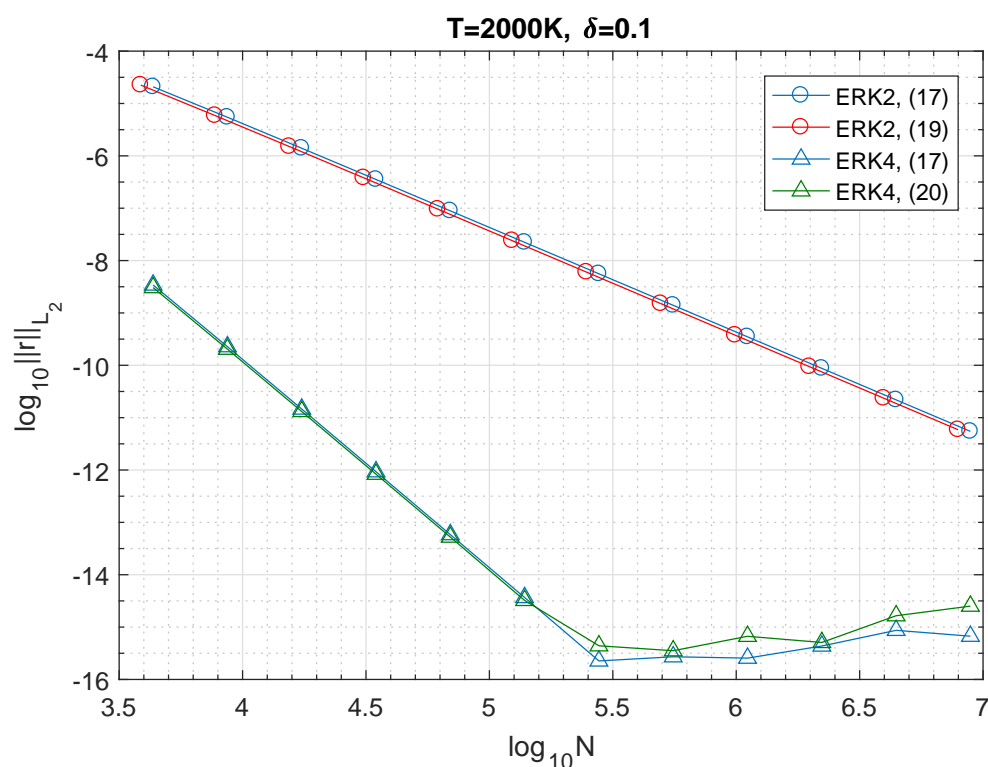
Рис. 10: Погрешности концентраций при различных способах вычисления кривизны (номер формулы указан в скобках), T = 2000 К.
