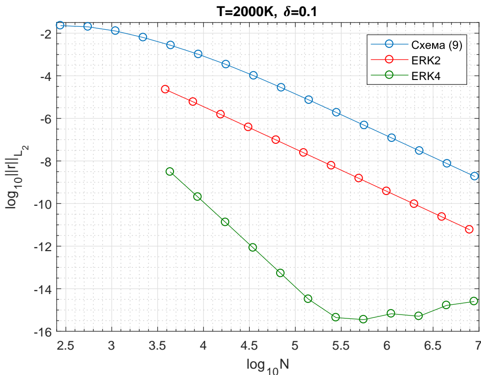
Рис. 4: Погрешности концентраций при сгущении сеток; T = 2000 К.
