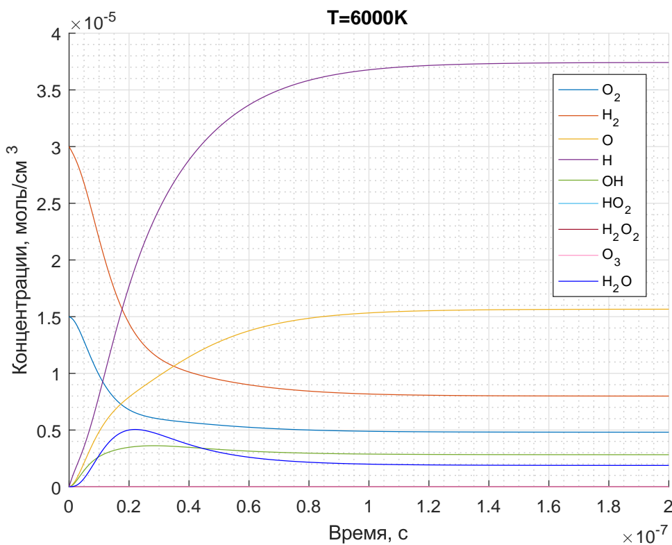
Рис. 2: Решение при температуре T = 6000 К.
