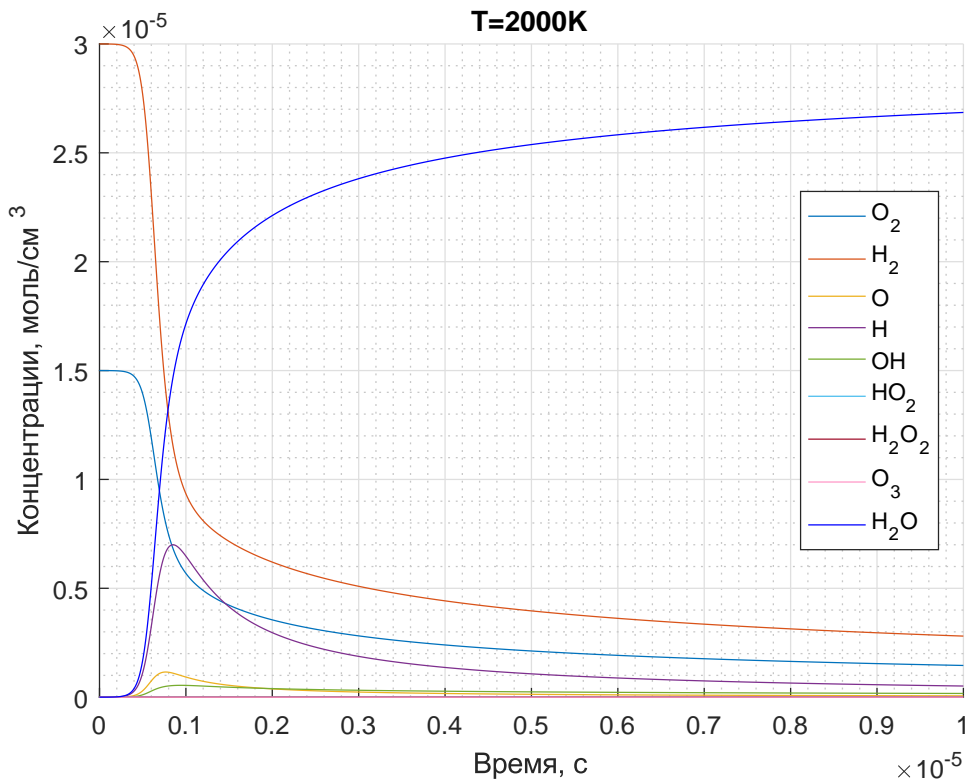
Рис. 1: Решение при температуре T = 2000 К.
