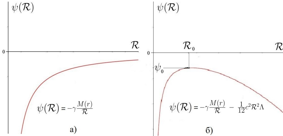
Рис. 1. Эффективный потенциал \psi(\mathcal{R}) с \Lambda = 0 (а) и \Lambda > 0 (б)
