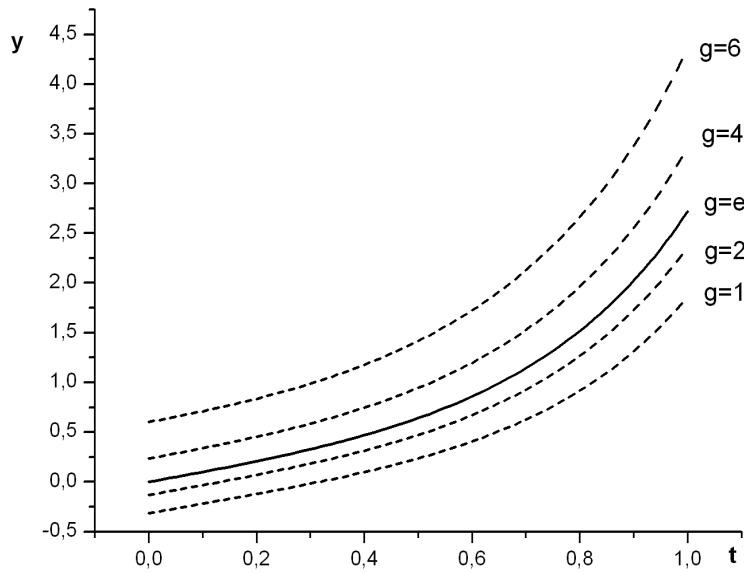
Рис. 1. Графики решений Примера 4 для различных значений g .
