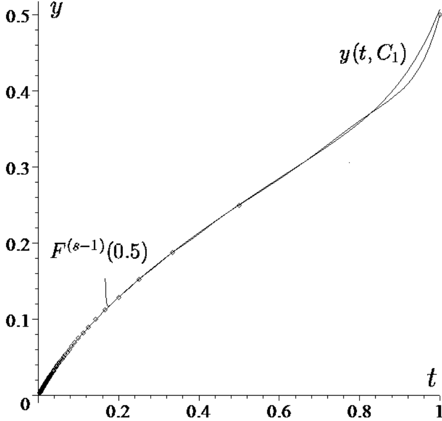
Рис 4. Асимптотика логистического отображения при 0 < z_0 < 1 .
