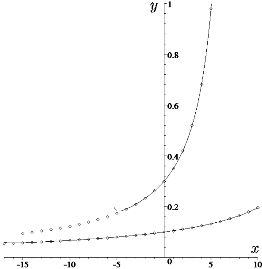
Рис 3. Непрерывные и дискретные итерации функции y = (\exp(z_0) - 1)^x .
