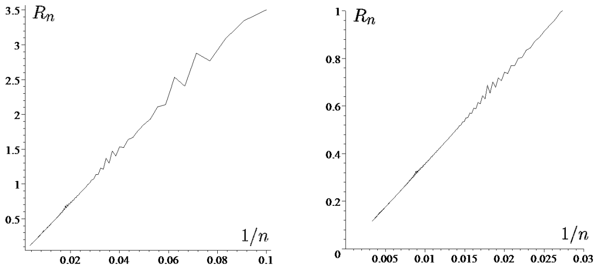
Рис. 1. Диаграмма роста коэффициентов формального ряда (\exp(z) - 1)^{(1/2)} .
