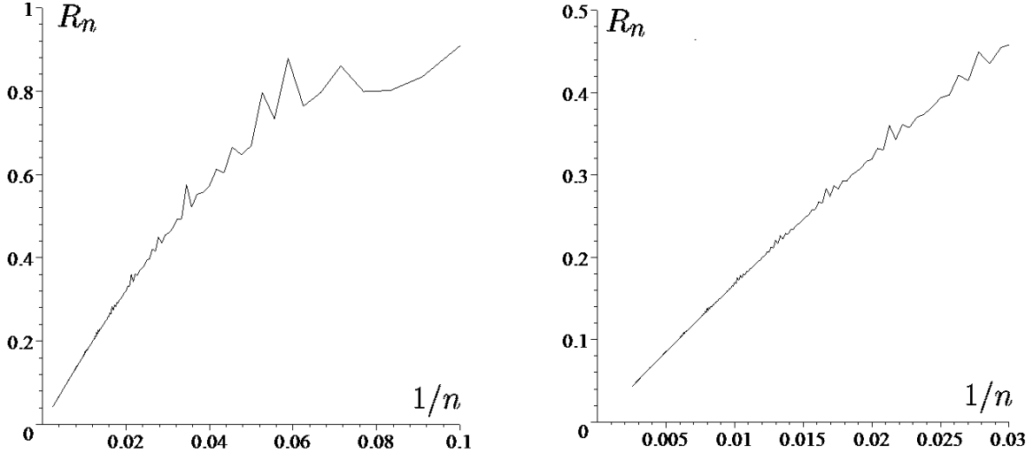
Рис. 2. Диаграмма роста коэффициентов формального ряда (z - z^2)^{(1/2)} .
