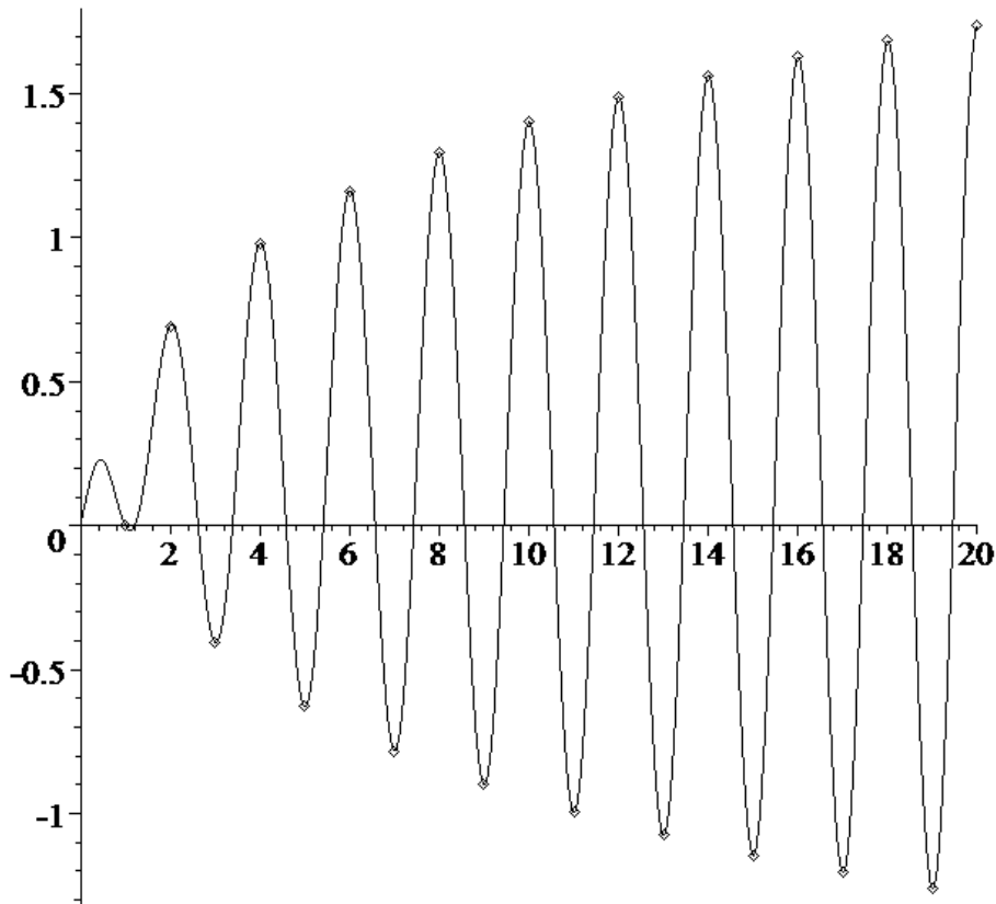
Рис 1. Частичные суммы ряда (29) и их интерполяция.
