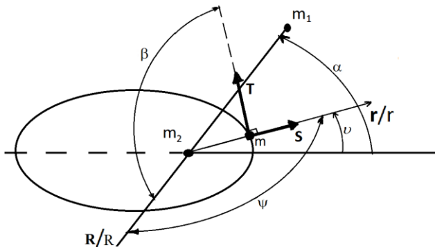
Рис. 9.1. Движение КА в поле двух притягивающих центров
