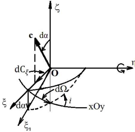
Рис. 6.4. Связь между элементарным приращением dc_{\xi} и элементарным поворотом d\Omega
