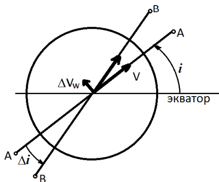
Рис. 10.1. Маневр КА над экватором при u = 0
